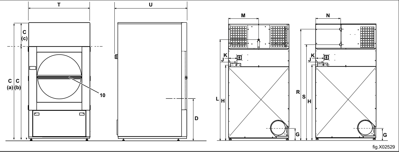
10 otwór drzwiczek z drzwiczkami przesuwными, \varnothing 940 mm
